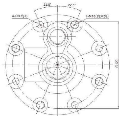
K向视图
